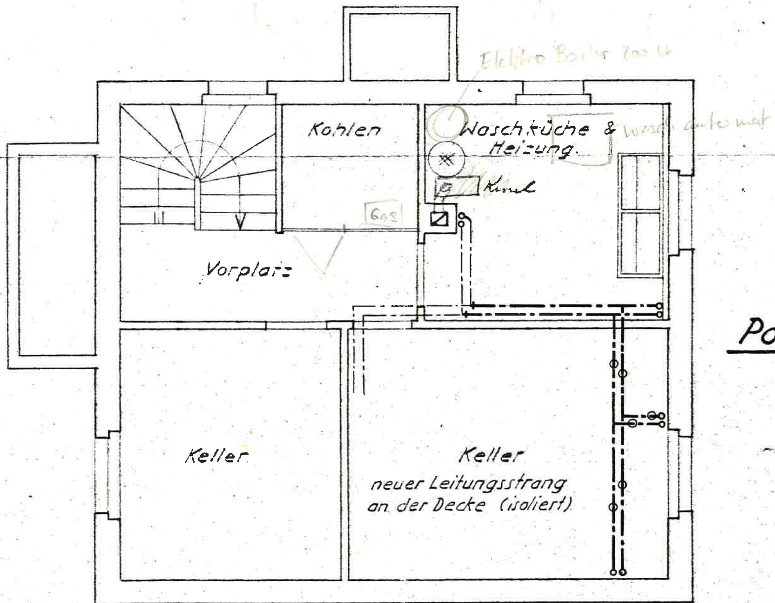
Keller-Grundriss.
