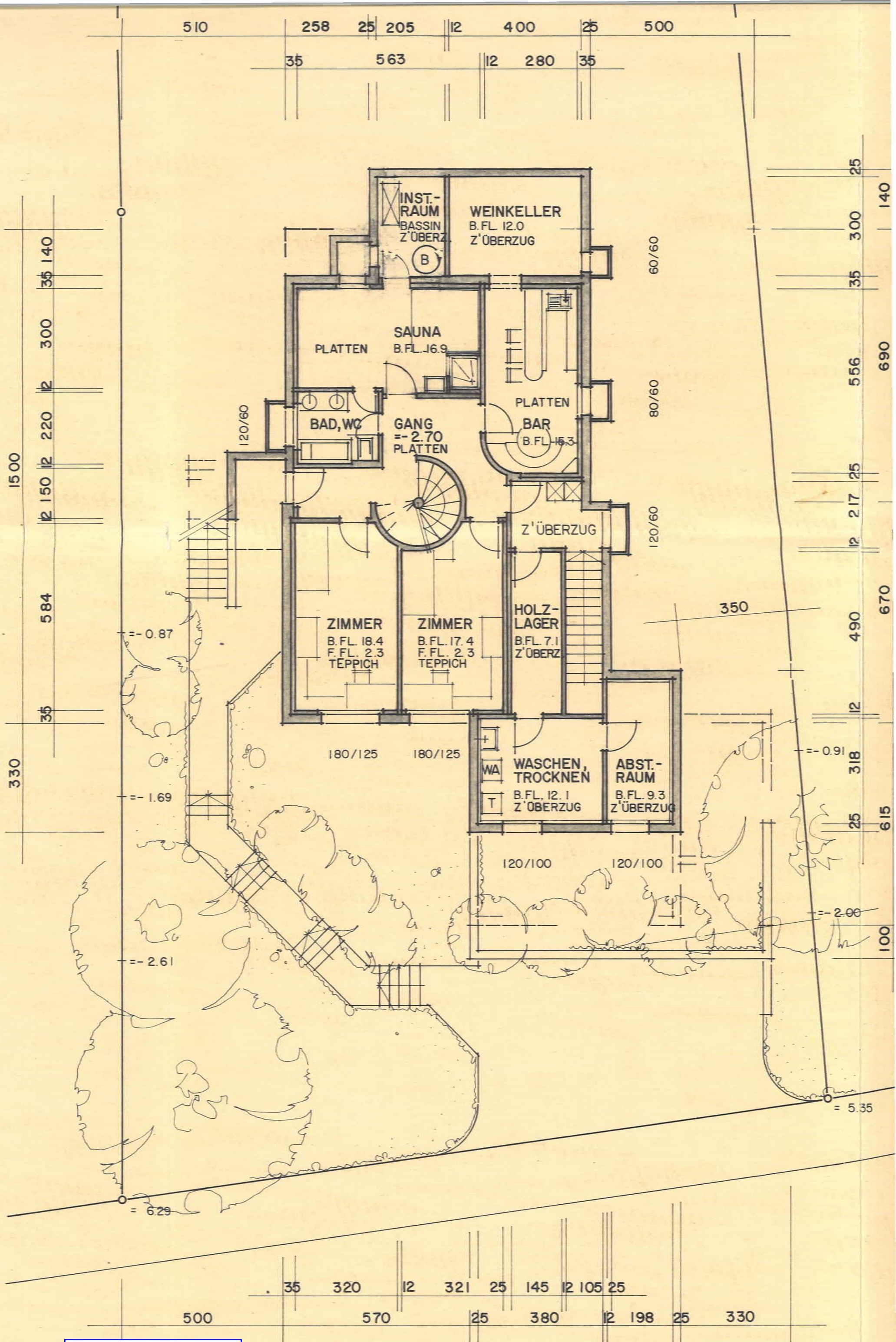
Untergeschoss
