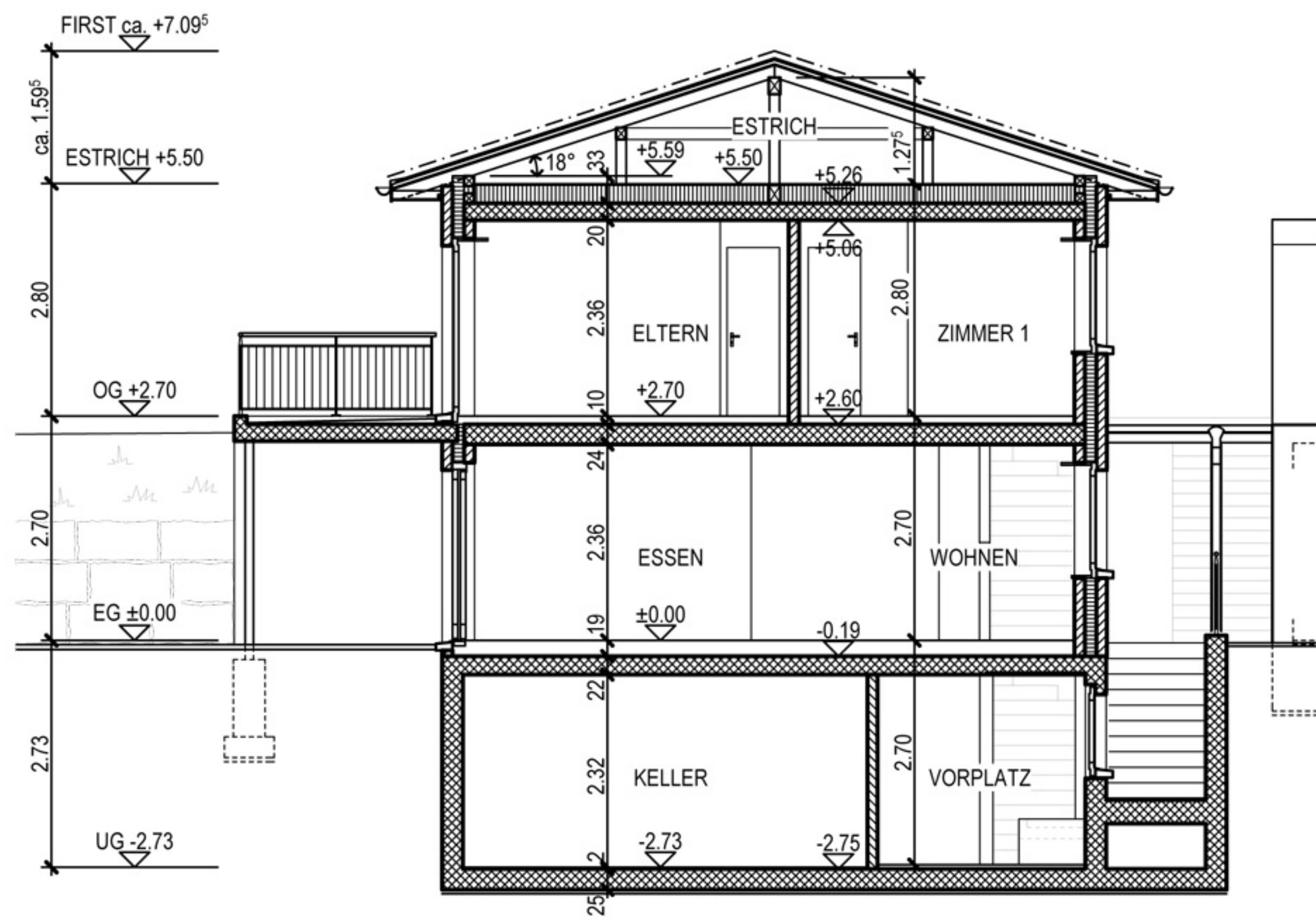
QUERSCHNITT
