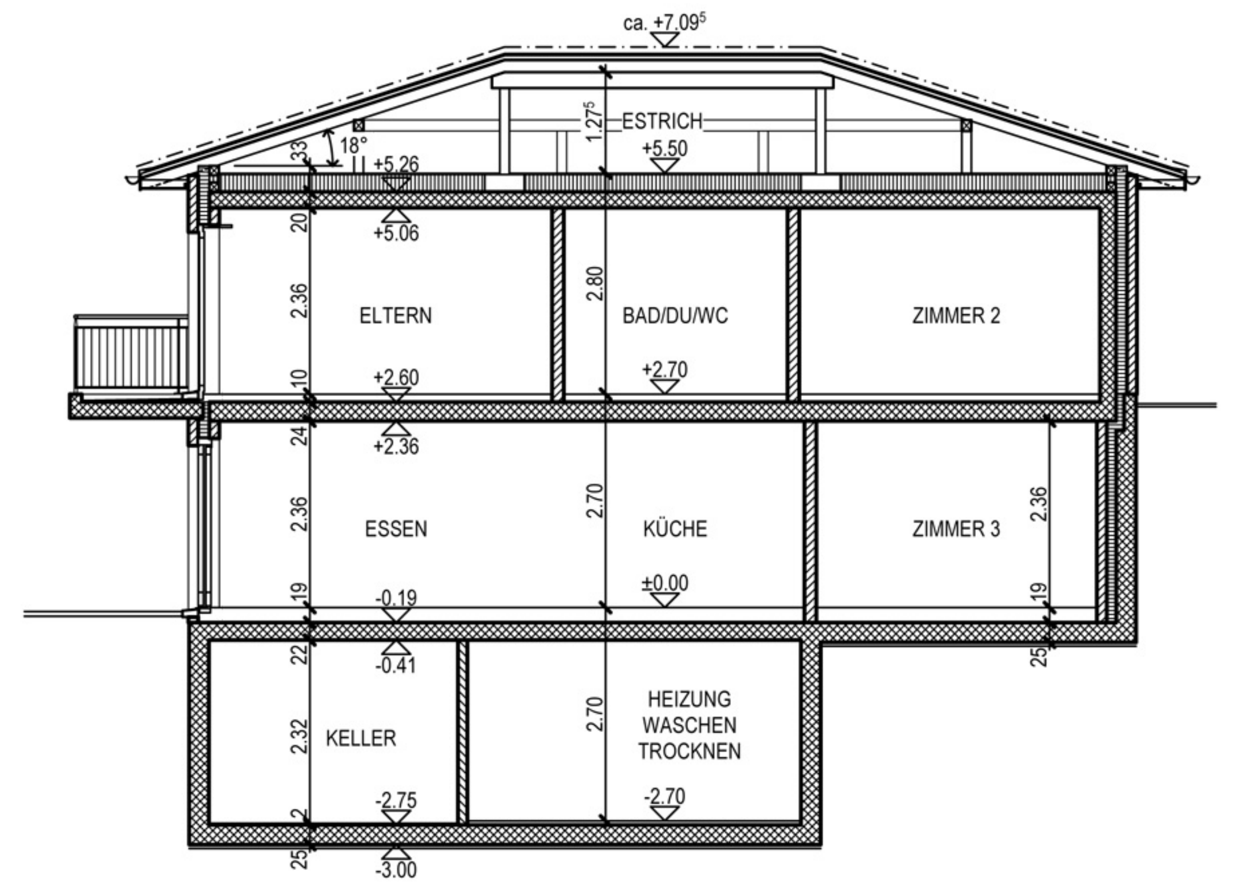
LÄNGSSCHNITT
