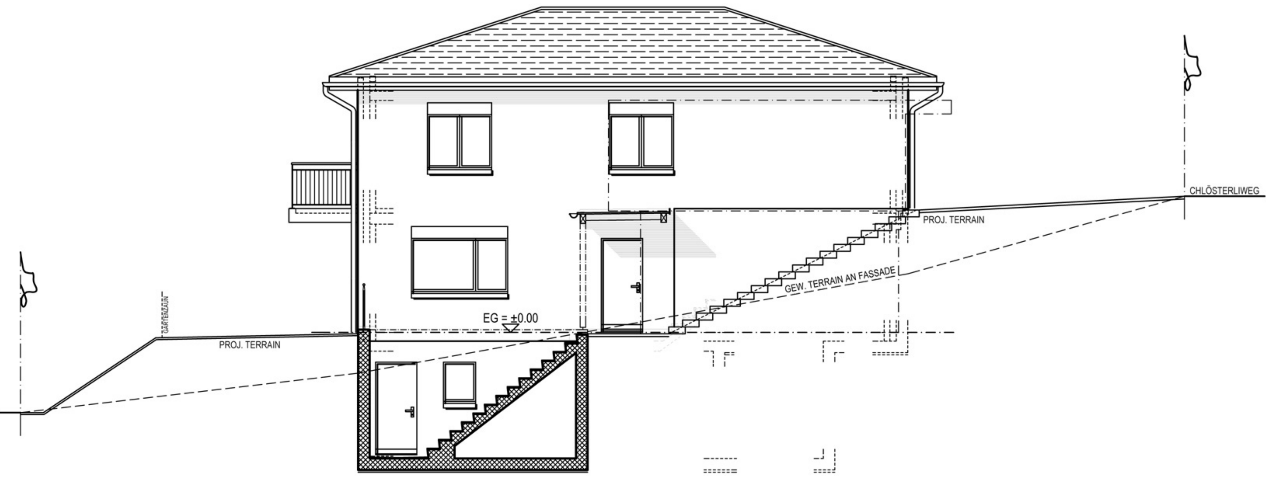
NORDOSTANSICHT
