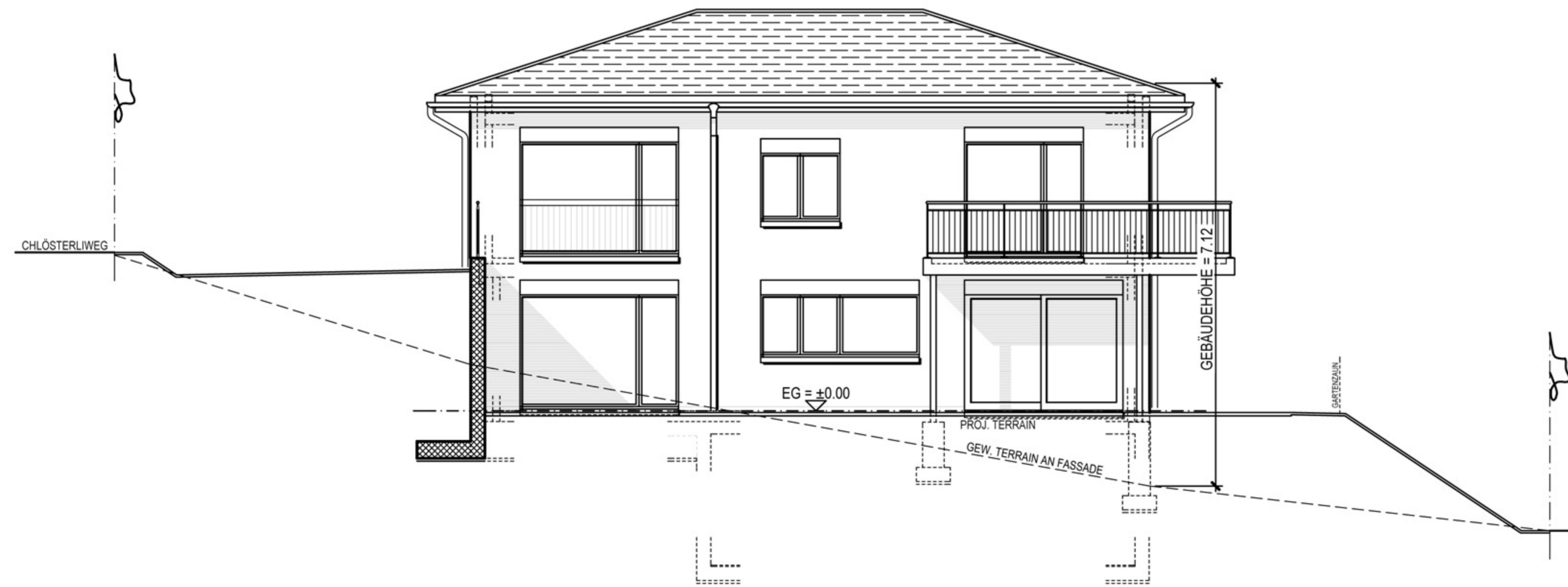
SÜDWESTANSICHT
