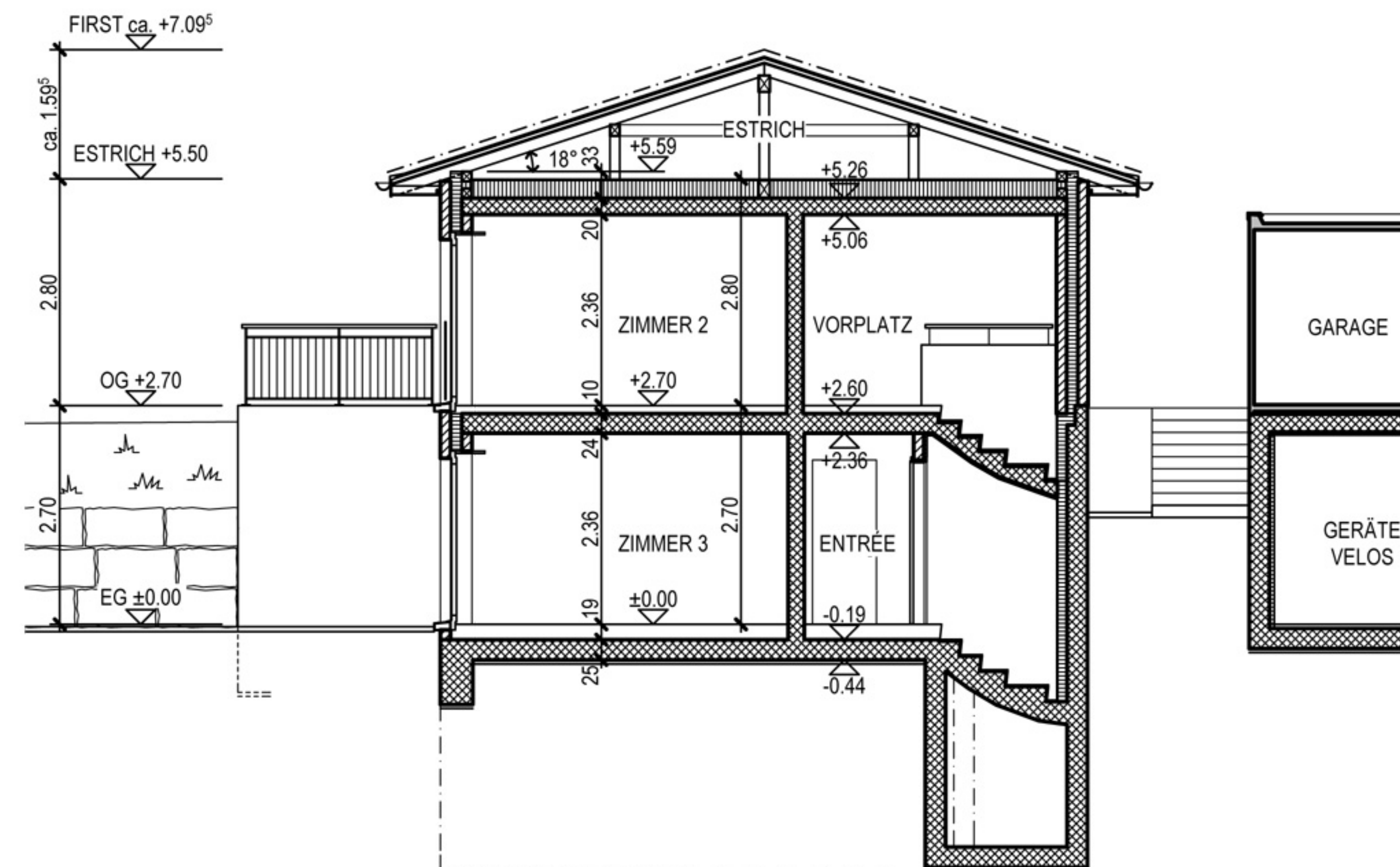
QUERSCHNITT TREPPE
