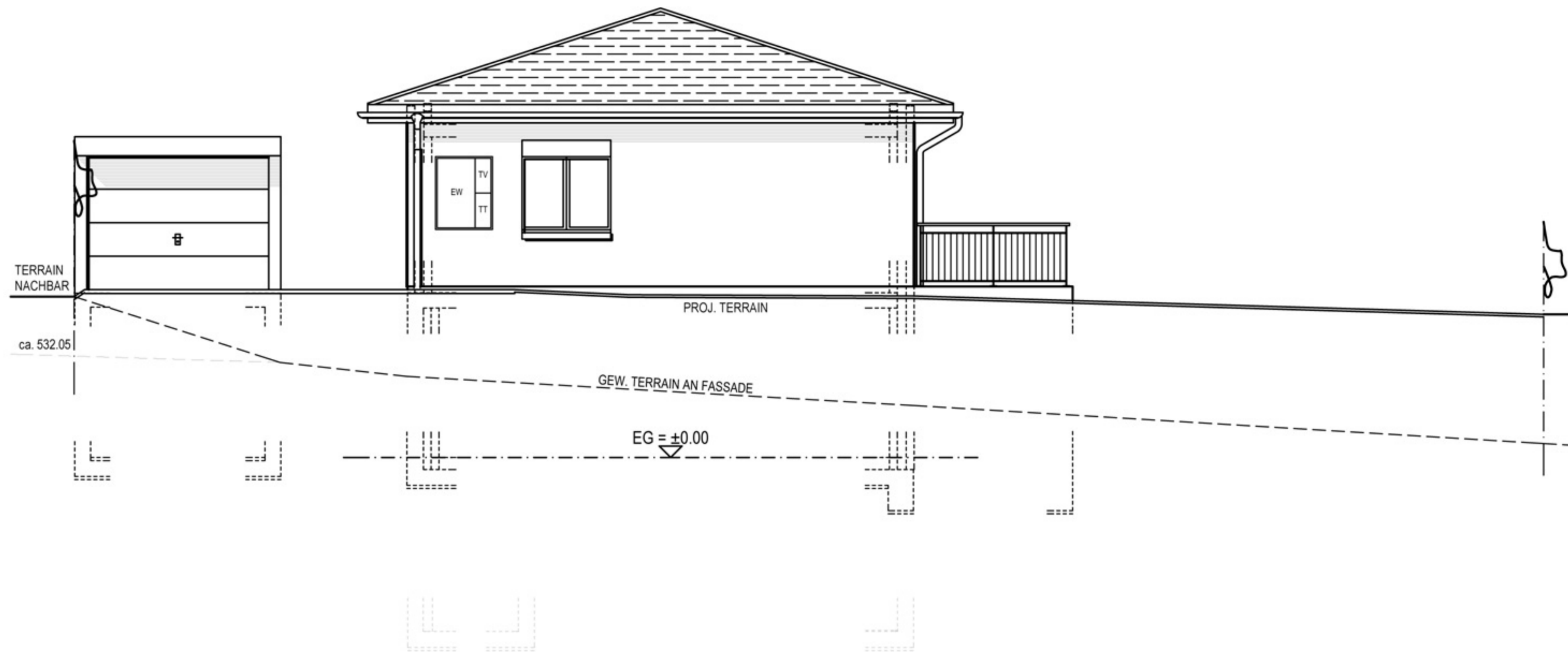
NORDWESTANSICHT
